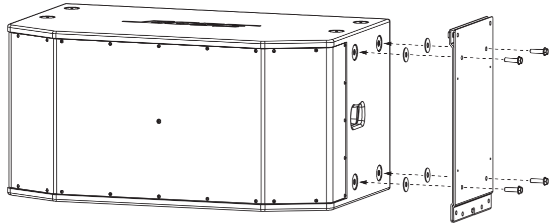
図2. 付属のボルトを使用してのサイドプレート取り付け
