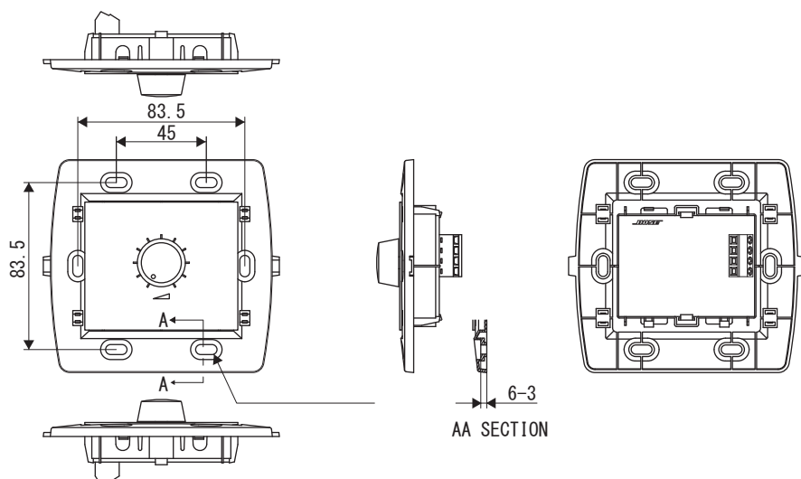
フロントパネル取外し時
